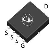
PDFN5x6
